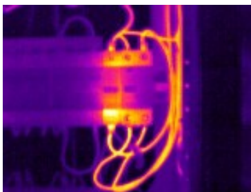
1. Kép http:// Hőkamerás felvétel az elektromos berendezés túlmelegedéséről
